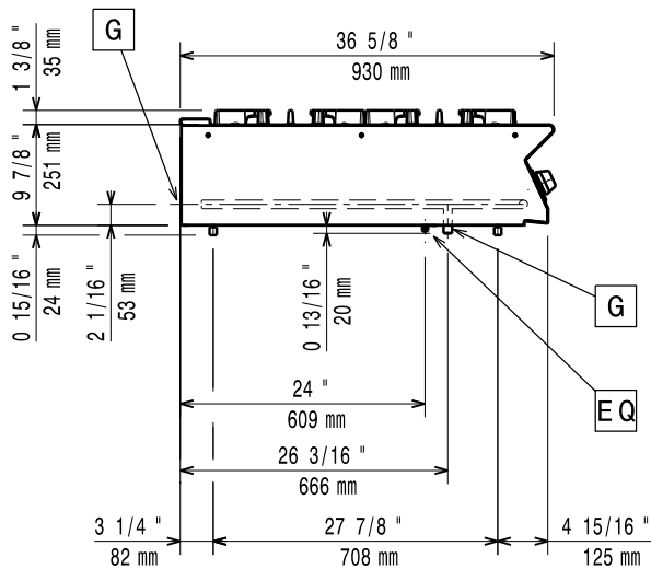
侧视
