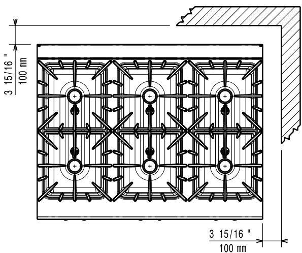
俯视
